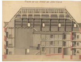
Coupe d'une salle de spectacle, 1777
