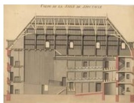
Coupe d'une salle de spectacle, 1777
